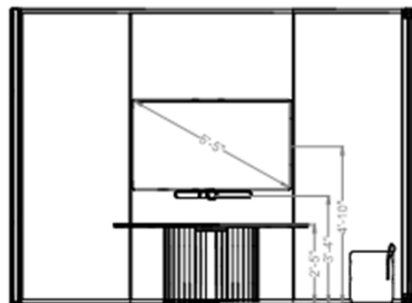
COUPE 3 | ELEVATION
